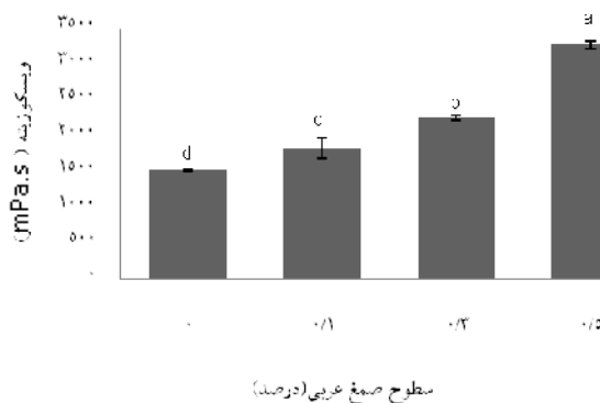
شکل ۴ اثر غلظت‌های مختلف صمغ عربی بر ویسکوزیته ظاهری مخلوط ماست منجمد (rpm=۷۰ و دمای ۵°C)
