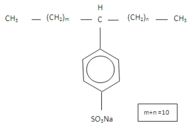
شکل ۱: ساختار شیمیایی LAS (همولوگ C 13 )
