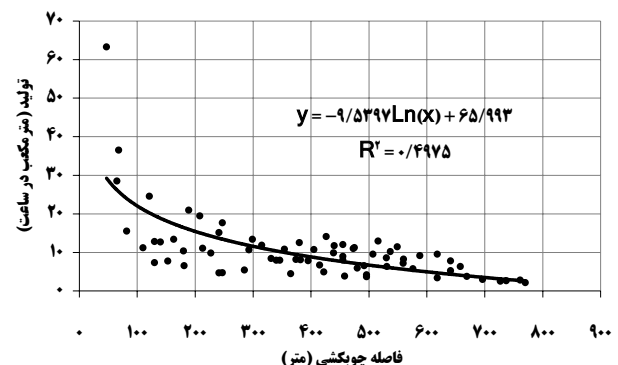
شکل ۱- تغییرات تولید چوبکشی در روش گرده‌بینة کوتاه در ارتباط با فاصله حمل
