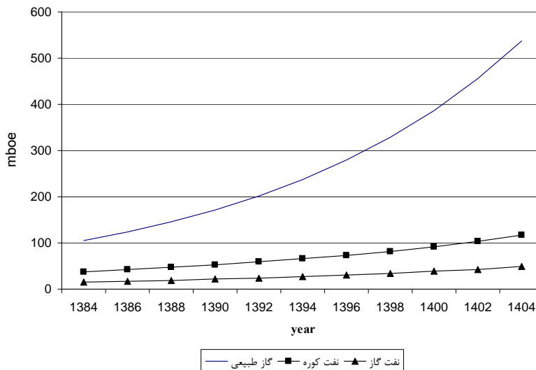
شکل ۵- محاسبه‌ی سوخت‌های فسیلی مورد نیاز برای تولید انرژی الکتریکی (۱۳۸۴-۱۴۰۴)، با در نظر گرفتن رشد مصارف نهایی
