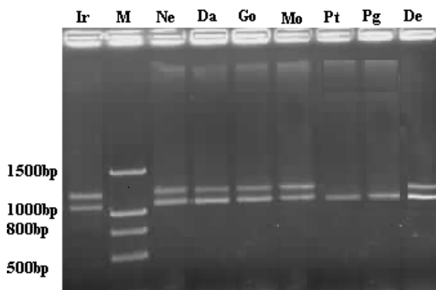
شکل(۲) نقوش الکتروفورزی محصولات PCR ناحیه IGS1 شش جدایه P. striiformis f.sp. tritici و دو شاهد Pt: Puccinia triticina
