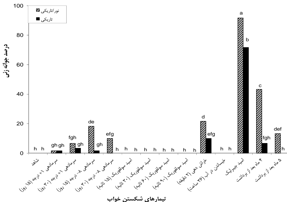
شکل ۲- تأثیر تیمارهای مختلف شکستن خواب بر جوانه‌زنی بذور شب‌بوی صحرائی بیمار شده در دمای 25/15^{\circ}\text{C} با دوره نوری ۱۲ ساعته در شرایط نور/تاریکی و تاریکی مداوم؛ ستون‌های فاقد حرف مشترک دارای اختلاف معنی‌دار بر اساس آزمون LSD در سطح ۵ درصد می‌باشند.
