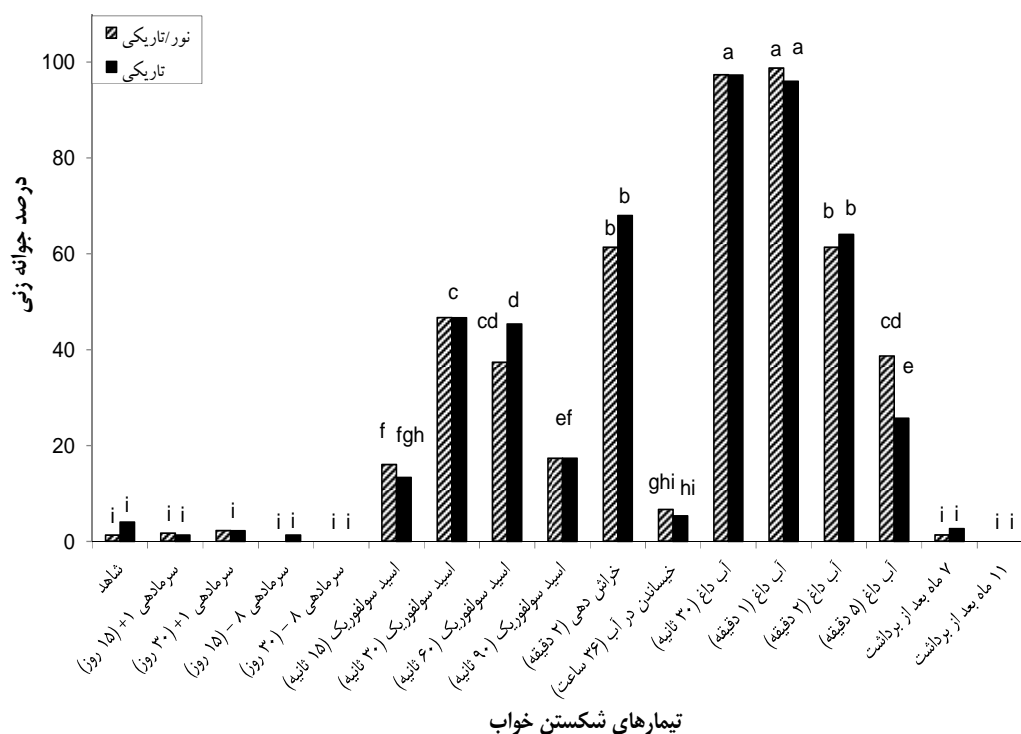
شکل ۱- تأثیر تیمارهای مختلف شکستن خواب بر جوانه زنی بذور سس شرقی تیمار شده در دمای ۲۵/۱۵ °C با دوره نوری ۱۲ ساعته در شرایط نور/تاریکی و تاریکی ستون‌های فاقد حرف مشترک دارای اختلاف معنی‌دار بر اساس آزمون LSD در سطح ۵ درصد می‌باشند.
