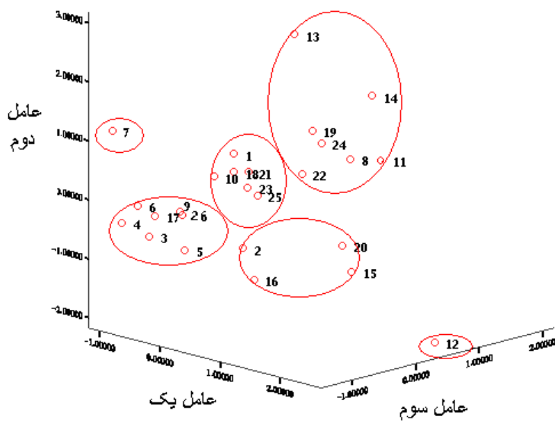
شکل (۳) دیاگرام تری پلات ۲۶ توده و رقم بایونه آلمانی با استفاده از فاکتورهای اصلی
