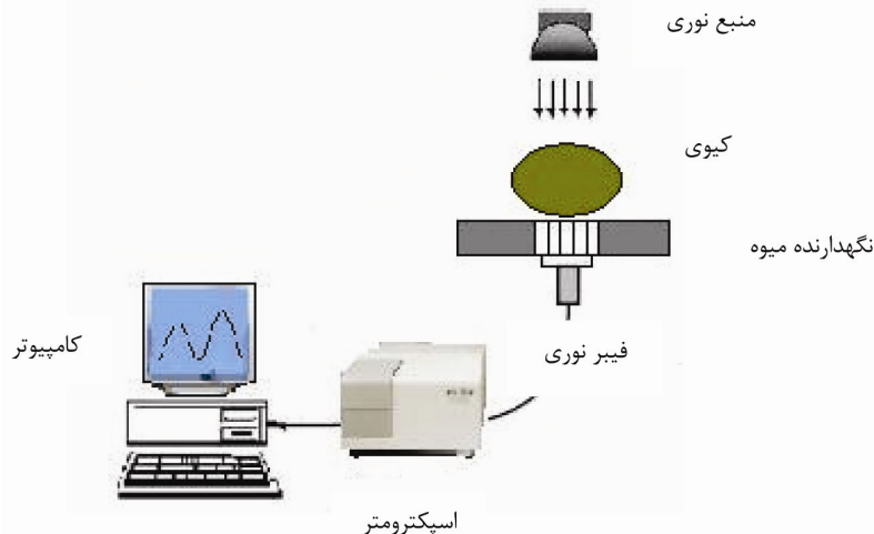
شکل (۱) نحوه ثبت طیف عبوری از کیوی در حالت افقی
