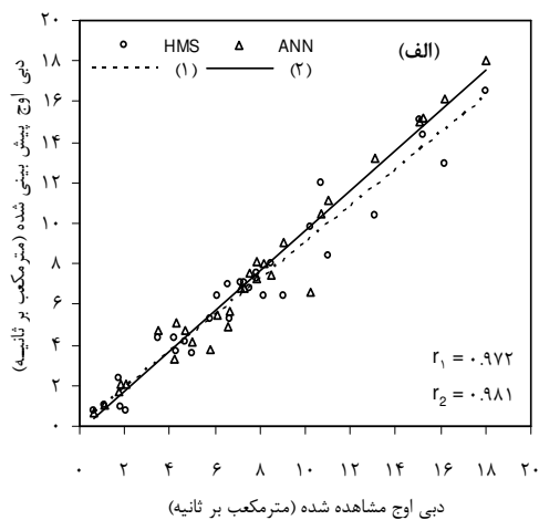
(شکل ۷) - برازش داده‌های دبی اوج (الف) و زمان اوج (ب) رواناب مشاهده شده و پیش‌بینی شده با شبکه عصبی مصنوعی (ANN) و سامانه مدل‌سازی آبخاکی (HMS) در حوزه آبریز کارده.
