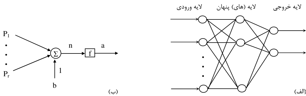
شکل ۱- (الف) ساختار کلی شبکه عصبی مصنوعی، (ب) نرون عصبی با تعداد ۲ ورودی و ۲ خروجی
