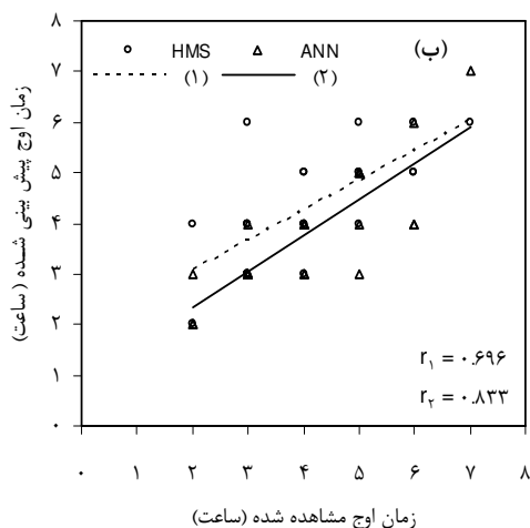
(شکل ۷) - برازش داده‌های دبی اوج (الف) و زمان اوج (ب) رواناب مشاهده شده و پیش‌بینی شده با شبکه عصبی مصنوعی (ANN) و سامانه مدل‌سازی آبخاکی (HMS) در حوزه آبریز کارده.
