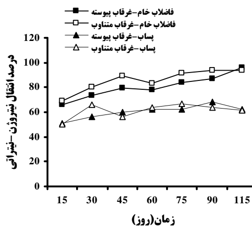
(شکل ۴) - درصد انتقال نیتروژن-نیتراتی از ستون‌های خاک به زه‌آب‌های خروجی در طول زمان
