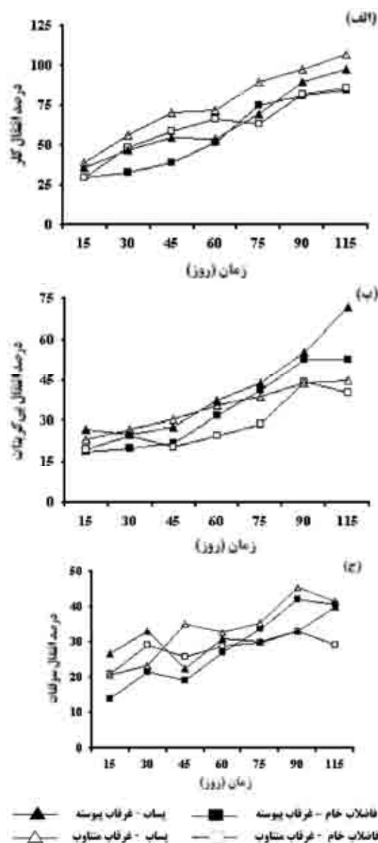
(شکل ۳) - درصد انتقال آنیون‌های محلول از ستون‌های خاک به زه‌آب‌های خروجی در طول زمان
