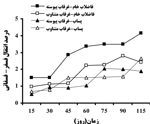
(شکل ۵) - درصد انتقال فسفر-فسفات‌های از ستون‌های خاک به زه‌آب‌های خروجی در طول زمان
