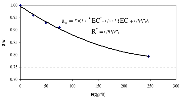
(شکل ۲) - رابطه‌ی درجه ۲ بین a_w با EC
