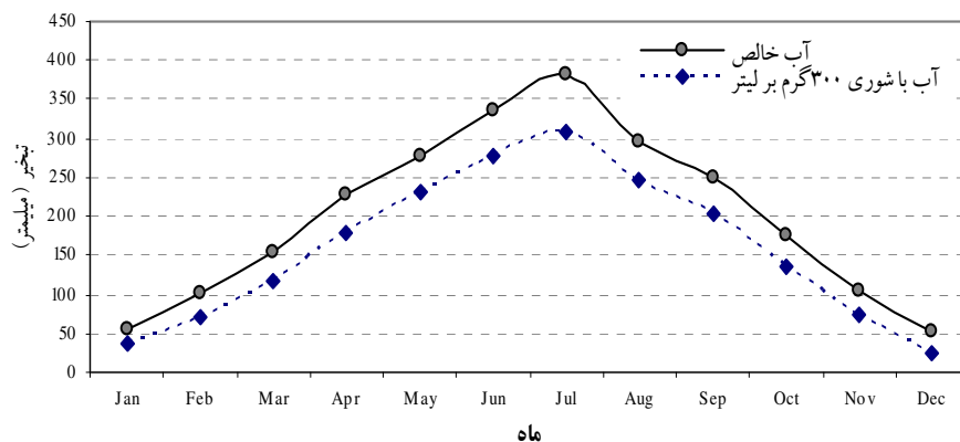
(شکل ۳) - میزان تبخیر ماهیانه برای آب خالص و آب با شوری ۳۰۰ گرم بر لیتر
