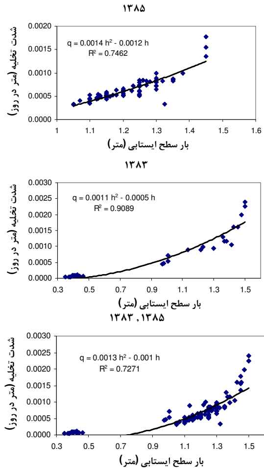
(شکل ۱۱) - رابطه دبی زهکش در مقابل بار سطح ایستابی برای چهار ماه سال ۱۳۸۵، سه ماه سال ۱۳۸۳ و کل داده‌های دو سال
