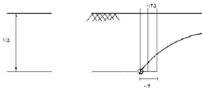
(شکل ۲) - محل نصب پیزومترها در مجاورت زهکش S3PD15 (ابعاد بر حسب متر)
