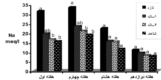
(نمودار ۹) - مقایسه اثر انواع SMC در زمان‌های مختلف در مقدار سدیم محلول آبشویی خاک
