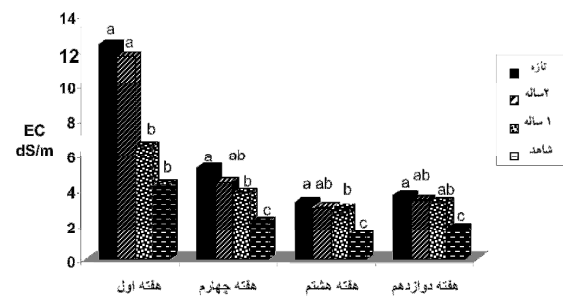
(نمودار ۸) - مقایسه اثر انواع SMC بر تغییرات EC محلول آبشویی خاک
