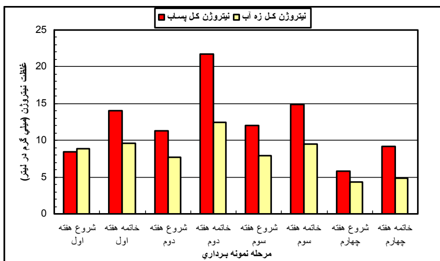
(شکل ۲) - میزان نیتروژن ورودی و خروجی سیستم تغذیه مصنوعی، در روش غرقابی - خشکی بلند مدت
