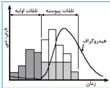
(شکل ۱) - نمایش شماتیک مدل تلفات اولیه - پیوسته با نرخ ثابت (۹)
