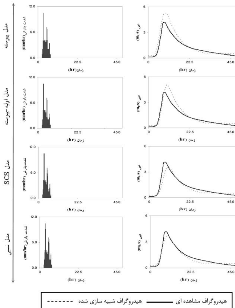
(شکل ۶ب) - مقایسه روش‌های تلفات باران در شبیه‌سازی هیدروگراف سیل در مرحله واسنجی (واقع در رگباری ۱۶/۸/۶۶)
