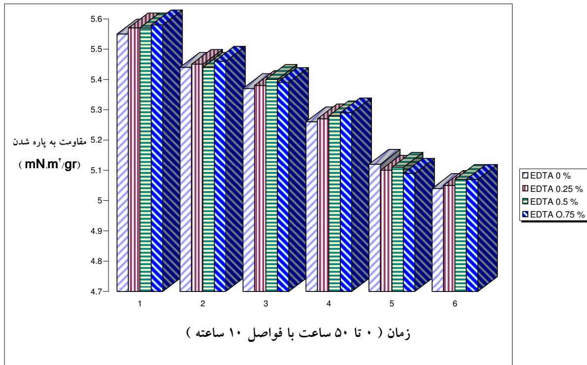
نمودار 2- تأثیر زمان و غلظت EDTA بر میزان شاخص مقاومت به پاره شدن کاغذ ساخته شده از خمیر اکالیپتوس
