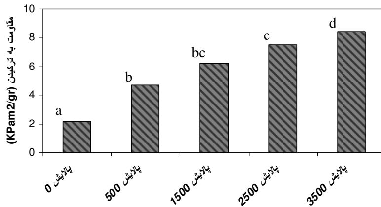
شکل 4- تأثیر شدت پالایش بر مقاومت به ترکیدن کاغذ حاصل از چوب اکالیپتوس کاملدولنسیس
