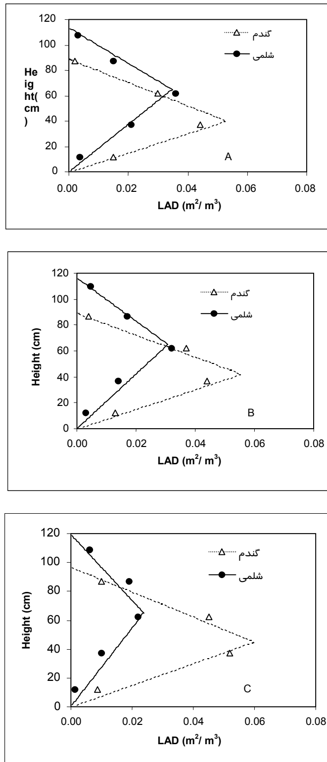
نمودار ۲- توزیع عمودی سطح برگ گندم و شلمی در ۱۸۰ روز پس از کاشت در تراکم های ۳۰۰ (A)، ۴۵۰ (B) و ۶۰۰ (C) بوته گندم در متر مربع در بالاترین تراکم شلمی ( 32 p/m^2 )
