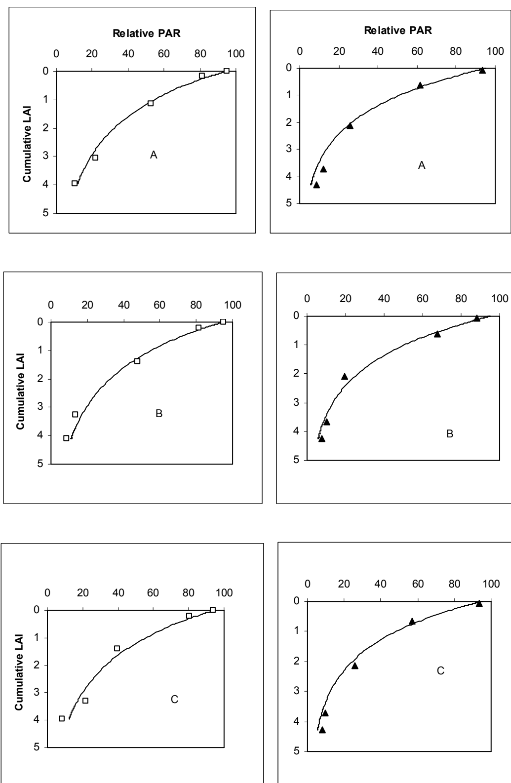
نمودار ۳- خاموشی نور در کانوپی مخلوط گندم و یولاف (سمت چپ)، گندم و شلمی (سمت راست) در تراکم‌های ۳۰۰ (A)، ۴۵۰ (B) و ۶۰۰ (C) بوته گندم در مترمربع در بالاترین تراکم علف هرز
