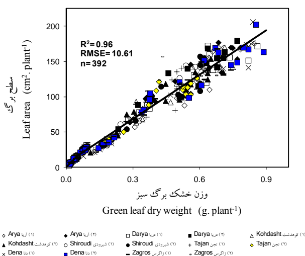
شکل ۴- برازش مدل رگرسیون دوتکه‌ای بین سطح برگ و وزن خشک برگ سبز در ارقام گندم و دو شرایط دیم و آبی (۱) و (۲) (داده‌های کل آزمایش). خط پیوسته نشان‌دهنده برازش رابطه ۶ به داده‌های کل آزمایش می‌باشد
