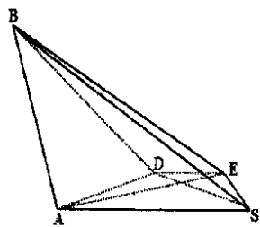
شکل ۱- ارتباط ژنومی میان پنج ژنوم اصلی طایفه گندمیان Fig.1. Genomic relationships among five basic genomes of triticeae tribe
