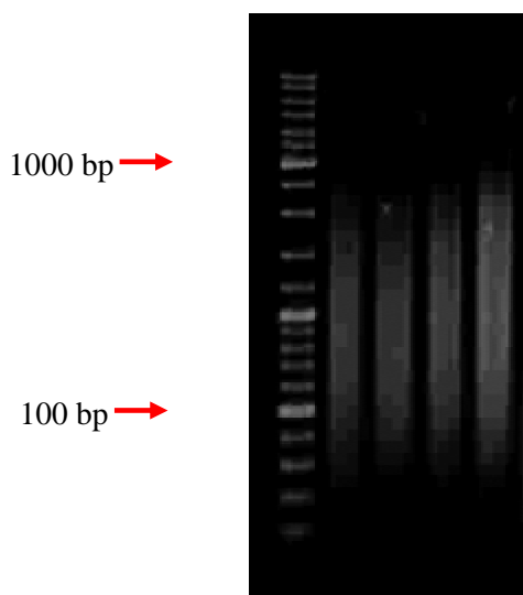
شکل ۲- کنترل طول 200 تا 1000 جفت بازی قطعات توالی دی.ان.ای مسدود کننده گندم بهاره چینی
