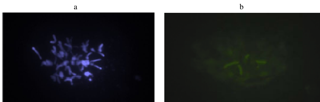
شکل ۴- دورگ‌گیری دی.ان.ای ژنومی در محل در مرحله متافاز میتوزی سلول‌های ژنوتیپ جدید و احتمالی تریتی‌پایرم ثانویه (NPSTIG) حاصل از تلاقی گندم نان (رقم نوید) با تریتی‌پایرم ترکیبی اولیه [لاین (Ka/b)(Cr/b)] با کاوشگر ژنومی گونه سودجینریا استیپی فولیا (نشاندار شده با بیوتین dUTP-۱۱) .a. فیلتر DAPI: تمام کروموزوم‌ها به رنگ آبی مشاهده می‌شوند. b. فیلتر فلورسئین ایزوتیوسیانات: تعداد ۴ کروموزوم دورگ‌گیری شده کاوشگر ژنومی S 1 با کروموزوم‌های همیولوگ ژنوم E b در NPSTIGs به رنگ سبز نورانی مشاهده می‌شوند (بزرگنمایی: ۴۰۰X)
