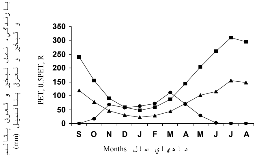
● PET : نصف تبخیر و تعرق پتانسیل 0.5PET : ■ تبخیر و تعرق پتانسیل (mm) : ▲ بارندگی R :
