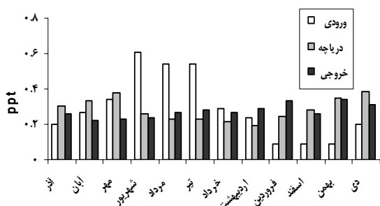
نمودار ۸- تغییرات غلظت نیترات در ورودی، خروجی و دریاچه پشت سد کرخه (۸۱-۸۲)
