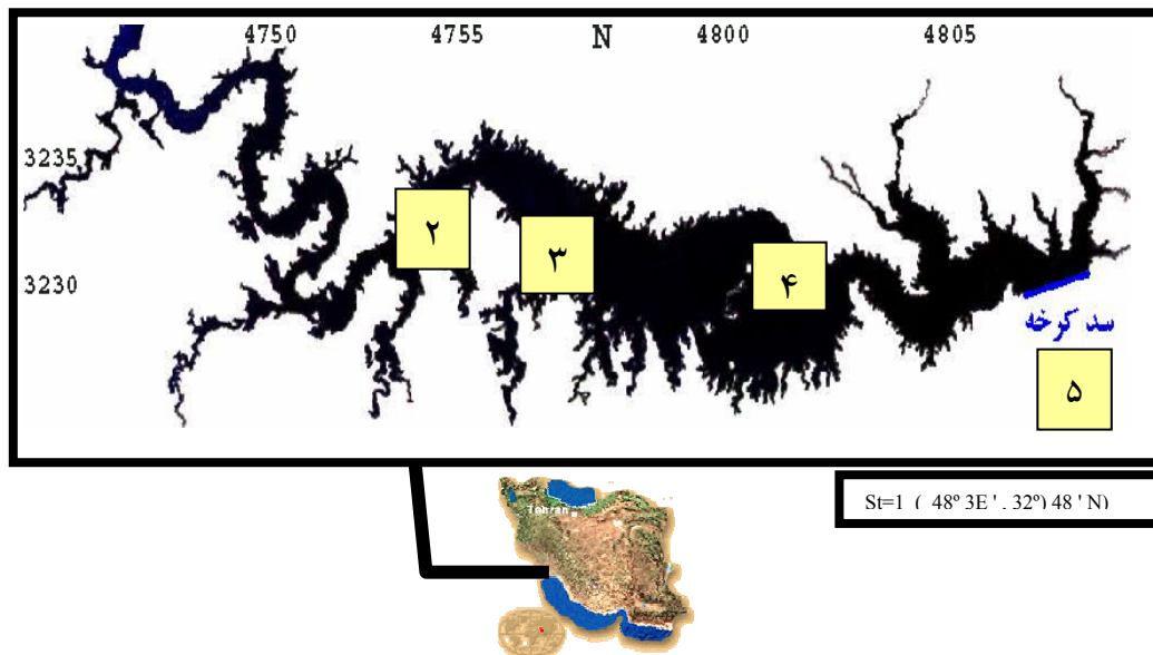
شکل ۱- نقشه ماهواره‌ای و موقعیت ایستگاه‌های نمونه برداری در دریاچه پشت سد کرخه
