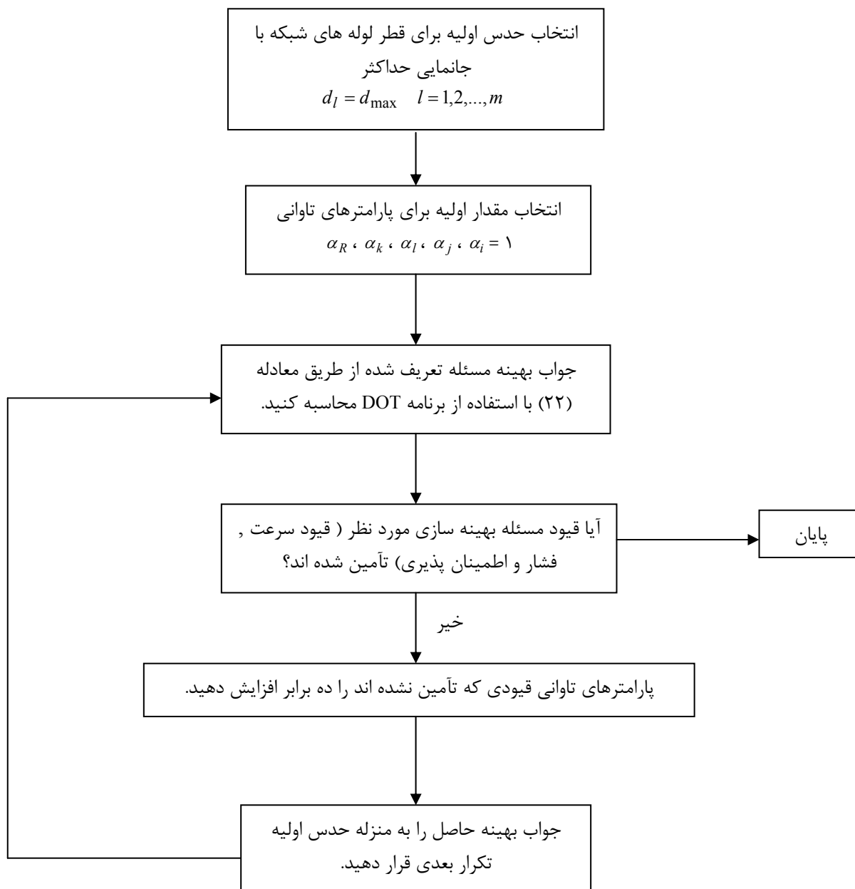
شکل ۴. نمودار شماتیک فرآیند بهینه سازی جانمایی
