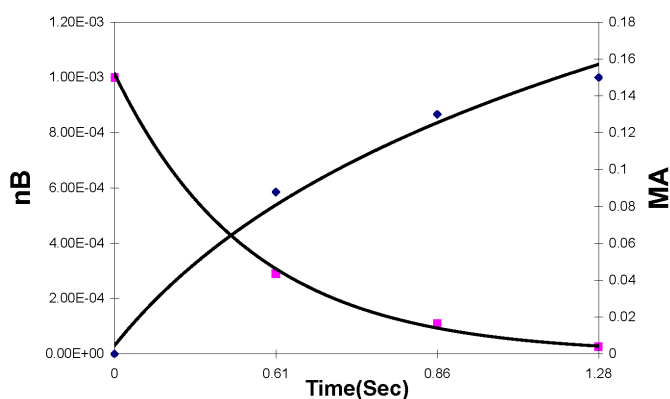
شکل ۷. غلظت نرمال بوتان ترکیب نشده و انیدرید مالئیک تولیدی در خروجی راکتور بر حسب زمان ماند گاز در راکتور، در دمای ۴۵۰ °C
