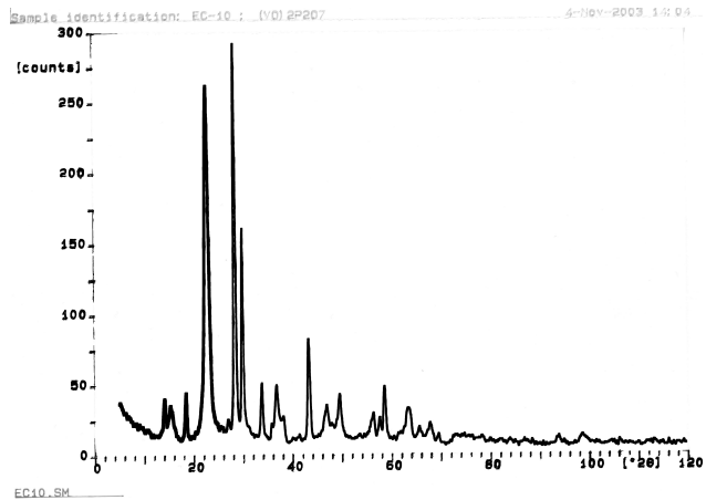
شکل ۱. الگوی پراش سنجی کاتالیزور ساخته شده
