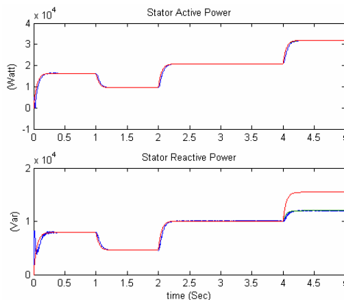
شکل ۱۴. تغییرات توان اکتیو و راکتیو ژنراتور با تغییر سرعت باد
