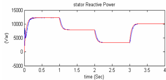
شکل ۹. تغییرات توان اکتیو و راکتیو ژنراتور با تغییر \cos \varphi_{ref}
