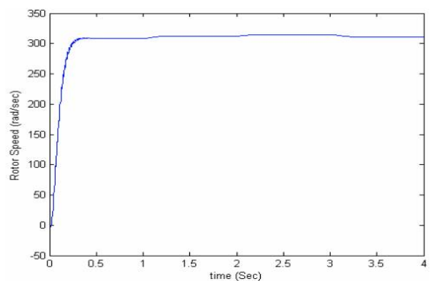
شکل ۱۱. تغییرات سرعت زاویه ای روتور با تغییر \cos \varphi_{ref}
