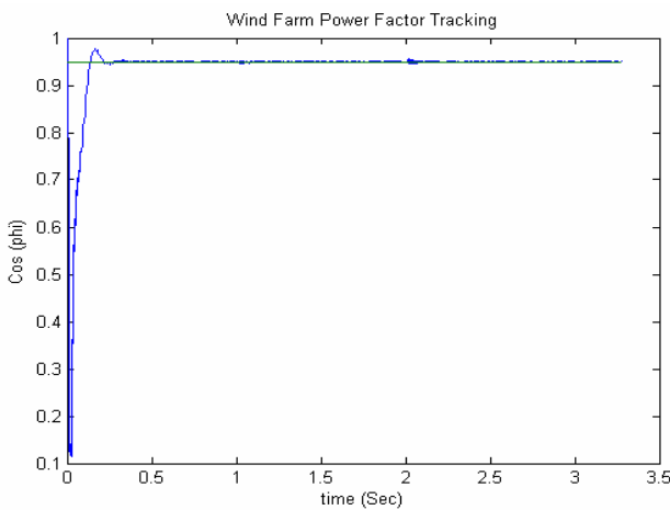
شکل ۱۹. ردیابی ضریب توان نیروگاه بادی با تغییر سرعت باد
