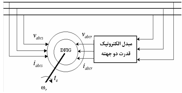
شکل ۲. ماشین القایی تغذیه شونده از دو طرف استاتور و روتور
