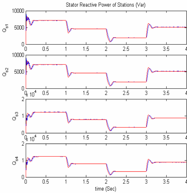
شکل ۱۸. ردیابی و تغییرات توان راکتیو هر ایستگاه
