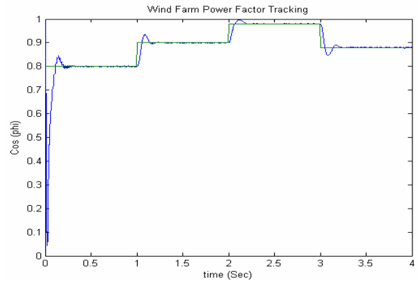
شکل ۱۶. ردیابی ضریب توان مرجع نیروگاه بادی
