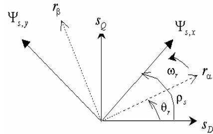
شکل ۳. دستگاههای مختصات دو محوری واقع بر استاتور، روتور و میدان دوار شار استاتور
