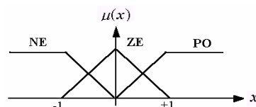
شکل ۶. مجموعه های فازی مربوط به متغیرهای فازی
