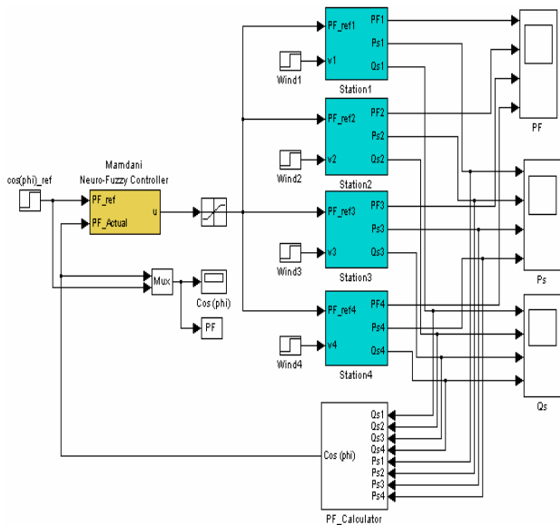
شکل ۱۵. توزیع توان راکتیو بین چهار ژنراتور DFIG
