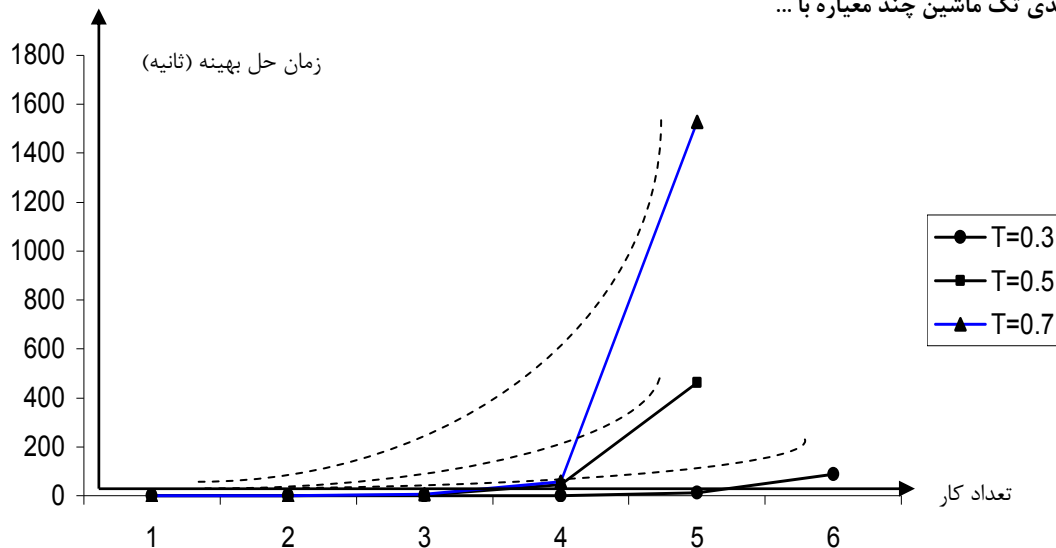
شکل ۱. تغییرات زمان حل بهینه بر حسب مقدار پارامتر T
