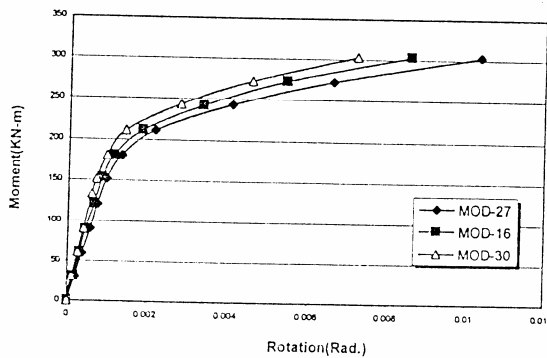
شکل ۱۵. منحنی لنگر- دوران با d متغیر (t=25, a=130)
