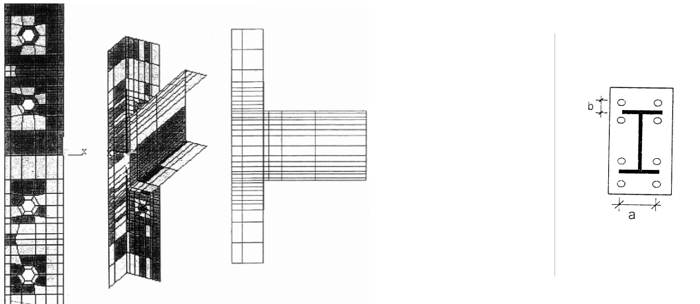
شکل ۱. مش بندی کل اتصال، صفحه انتهائی و مدل دو بعدی اتصال
