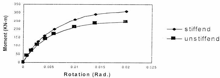
شکل ۱۷. مقایسه منحنی لنگر- دوران اتصال با ستون دارای سخت کننده و بدون آن
