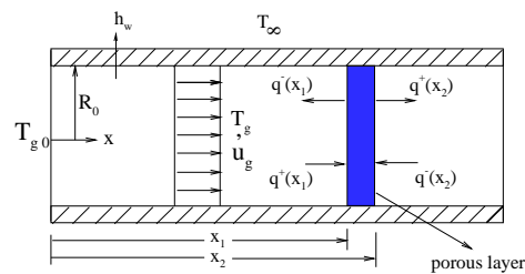
شکل ۱. نمایی از یک سیستم بازیافت انرژی
