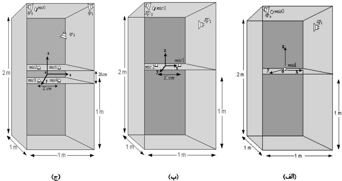
شکل ۱۱. آرایش میکروفن ها و بلندگوها در محفظه در سیستم ANC (الف) تک کاناله (ب) چند کاناله 1 \times 1 \times 2 و (ج) چند کاناله 1 \times 2 \times 4
