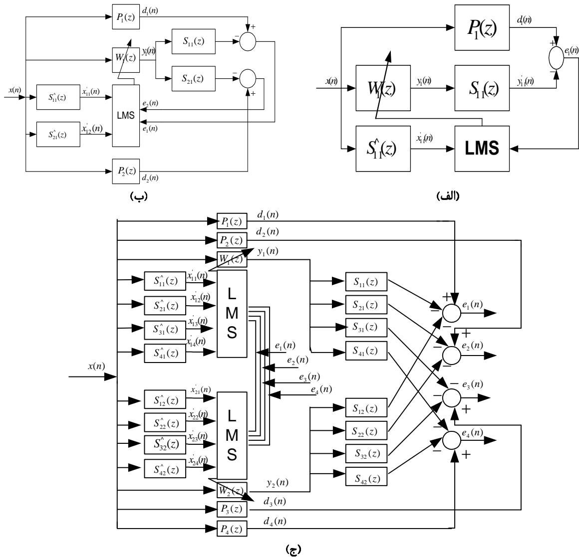
شکل ۱۳. جزئیات بلوک دیاگرام سیستمهای ANC پیاده سازی شده (الف) تک کاناله (ب) 1 \times 1 \times 2 و (ج) 1 \times 2 \times 4
