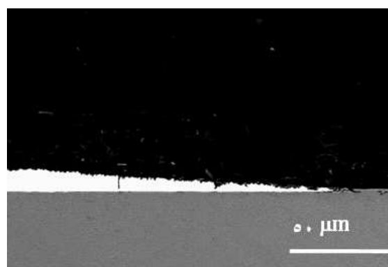
شکل ۱۲. تصویر SEM از مقطع عرضی اثر ساییش پوشش شکل ۱۱ پس از شکست (۱۰۰۰ متر مسافت لغزش)
