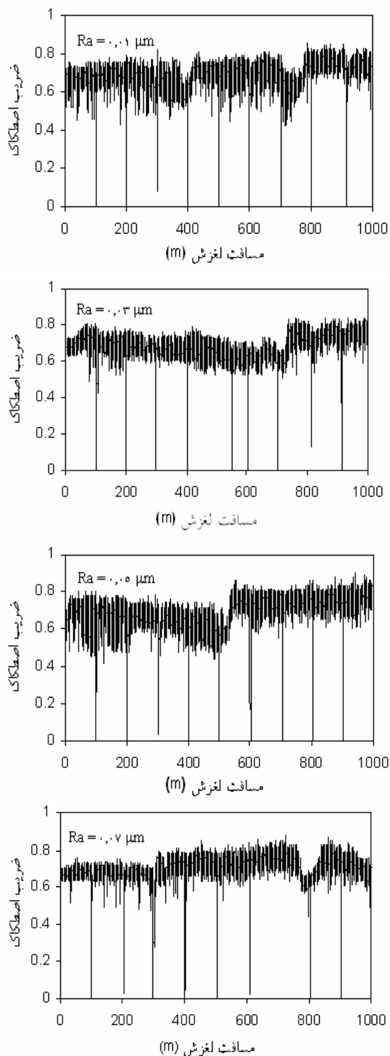
شکل ۱۴. تغییرات ضریب اصطکاک بر حسب مسافت لغزش برای پوششهای با زبری زیرلایه متفاوت تحت بار ۲ kgf و سرعت لغزشی ۰/۱ m/s
