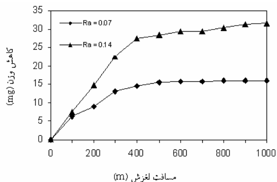
شکل ۵. منحنی مشخصه سایش پوششهایی که زبری زیرلایه آنها به روش الکتروشیمیایی ایجاد شده، تحت نیروی ۲ kgf و سرعت لغزش ۰/۱ m/s
