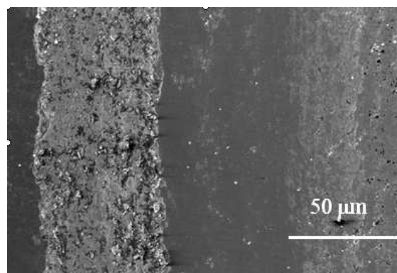
شکل ۱۱. تصویر SEM از سطح اثر ساییش پوشش با زبری زیر لایه ۰/۰۷ میکرون تحت نیروی ۵ kgf پس از ۱۰۰۰ متر مسافت لغزش (شکست پوشش اتفاق افتاده و زیر لایه نمایان شده است)
