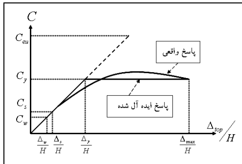
شکل ۱. منحنی پاسخ یک سازه متعارف [5]
