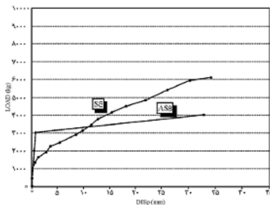
شکل ۷. منحنی‌های بار - تغییر مکان بر اساس نتایج آزمایش و تحلیل نمونه S8 (AS8 منحنی مربوط به تحلیل)
