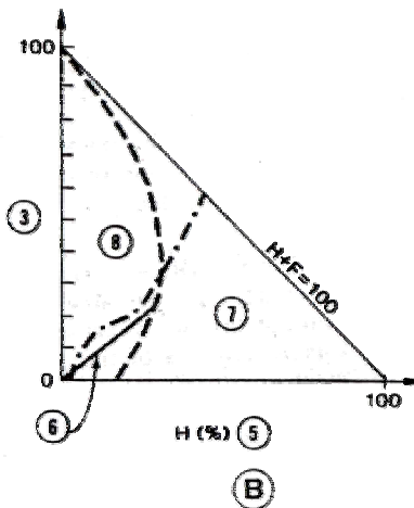
A: منحنی دانه‌بندی، B: منحنی شکل، 1: فیلتر شماره ۱، ناپایدار داخلی، 2: فیلتر شماره ۲، پایدار داخلی، 3: درصد وزنی ریزتر، 4: اندازه دانه‌ها (d)، 5: H، 6: مرز H=F ، 7: پایدار، 8: ناپایدار شکل ۲. طریقه رسم و تشخیص پایداری داخلی به روش کنی-لو [5]
