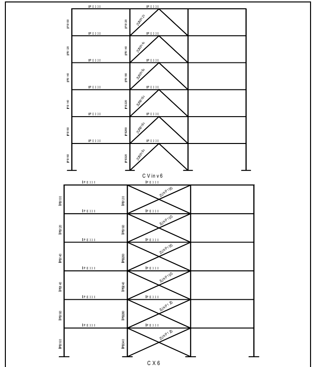
شکل ۳. مدل‌های شش طبقه طراحی شده بر اساس
