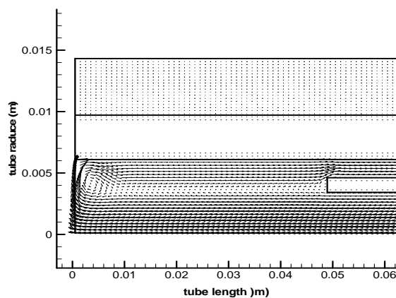
شکل ۱۶. بردارهای سرعت در کانال های سوخت و هوا در
