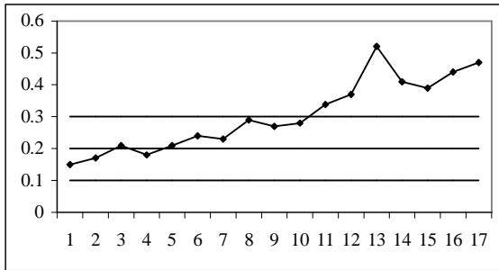
شکل ۱. روند صعودی در نمودار کنترل نسبت ارقام معیوب بدلیل فرسایش ابزار
