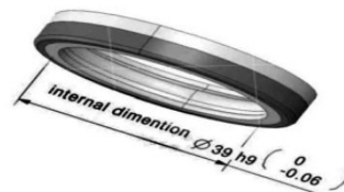
شکل ۲. قطر داخلی کاسه نم
