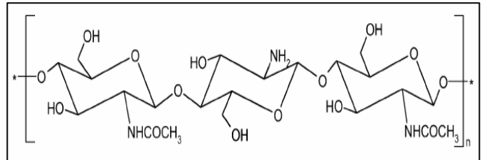
شکل ۱ ساختار کیتوزان
