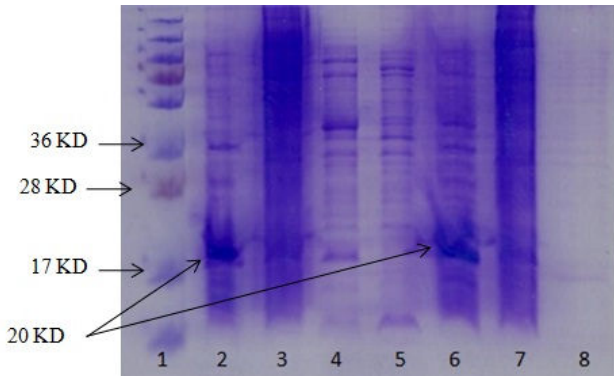
شکل ۲. الکتروفورز SDS-PAGE پروتئین های استخراج شده با سیاه زخم ستونها: (۱) نشانگر وزن مولکولی پروتئین، (۲) و (۳) بیان پروتئین مورد نظر با وزن مولکولی ۲۰ کیلوالتون
