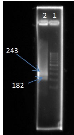
شکل ۱. الکتروفورز برش محصول PCR مربوط به ناحیه کربوکسیل انتهایی پروتئین PA با سیاه زخم روی ژل آگارز ۲ درصد. ۱. DNA ladder و ۲. باندهای ۱۸۲ و ۲۴۳ حاصل از برش آنزیمی توسط Eco57I (AclI)
