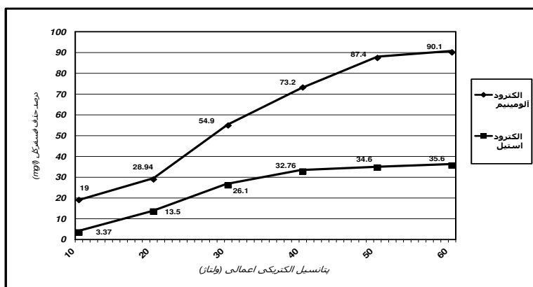
نمودار ۱: روند حذف الکتروشیمیایی فسفر کل نسبت به پتانسیل الکتریکی اعمالی با استفاده از الکتروود استیل، در مقایسه با الکتروود آلومینیومی
