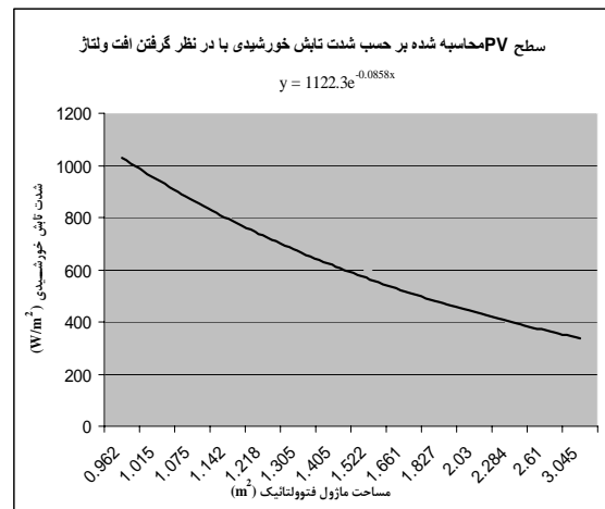
شکل ۳- منحنی تغییرات سطح ماژول فتوولتائیک بر حسب شدت تابش خورشیدی در سناریوی دوم
