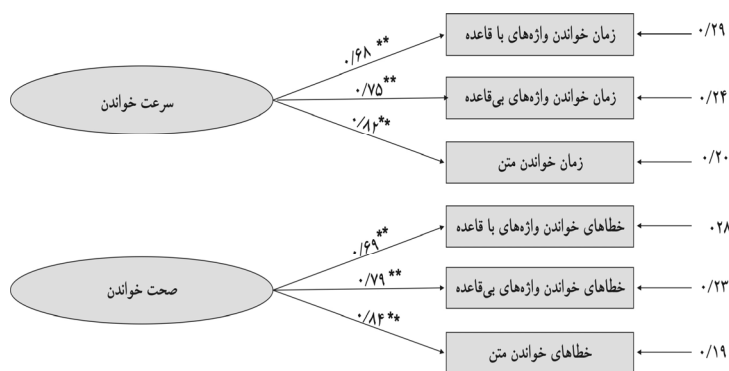
شکل ۲- مدل اندازه‌گیری متغیرهای نهفته درونزا در گروه یک زبانه عادی P < 0.01
