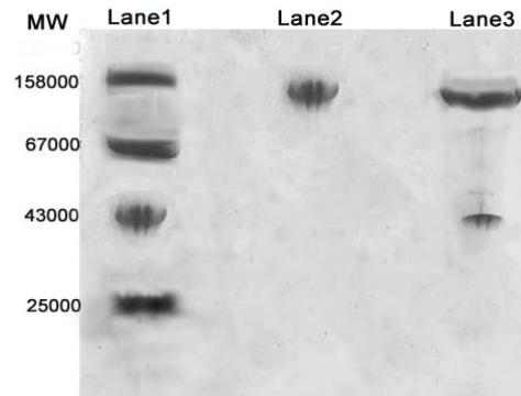
شکل ۳- الکتروفورز پلی آکرلامید در حضور سدیم دودسیل سولفات از فرآورده ^{99m}\text{Tc-PR81} با رنگ آمیزی کوماسی آبی. ستون اول: استانداردهای وزن مولکولی (MW)، ستون دوم: آنتی بادی PR81 دست نخورده، ستون سوم: فرآورده ^{99m}\text{Tc-PR81}
