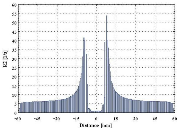
شکل ۴- R2 نقاط مختلف روی یک پروفایل عرضی همسطح چشمه سزیم در دوزیتر اول بر حسب فاصله از مرکز چشمه
