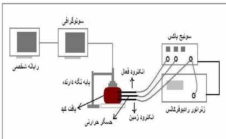
شکل ۱- چیدمان آزمون
