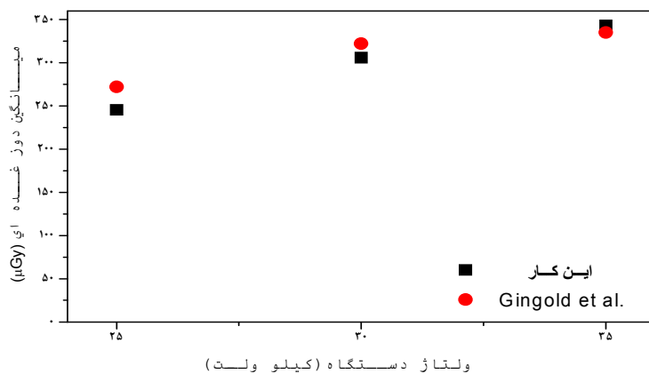
شکل ۵- مقایسه نتایج تجربی گینگلدوهمکارانش با نتایج حاصل از این پژوهش برای ضخامت پستان ۲ سانتی متر و ولتاژ ۲۵، ۳۰ و ۳۵ کیلو ولت و ضخامت نیم لایه-ها g=0.25 متناظر به ازای
