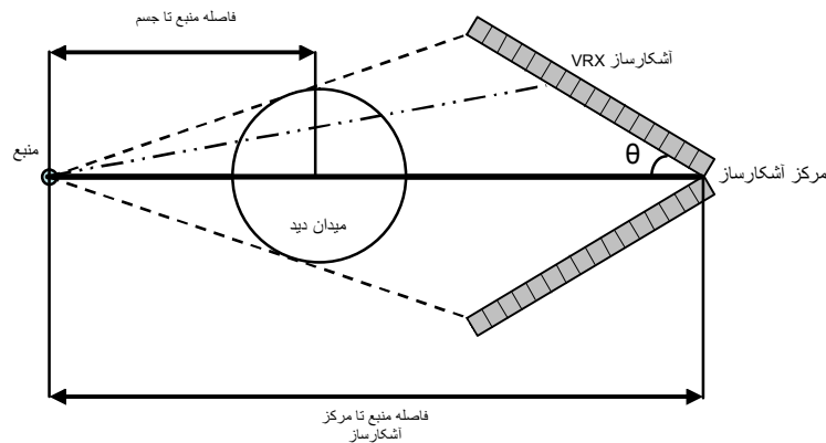
شکل ۱- طرحی از یک دستگاه سی تی
