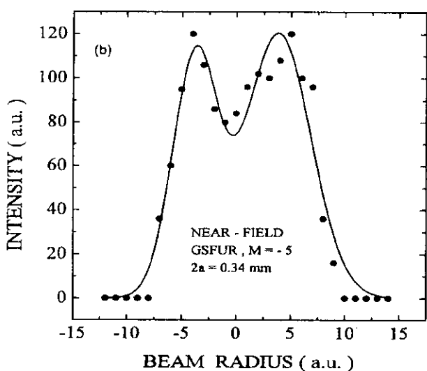
شکل ۵- نمونه‌ای از توزیع شدت میدان نزدیک، اندازه‌گیری با مشاهده فلورسان صفحه مشاهده و آشکار سازی به وسیله دوربین CCD بوده است.
