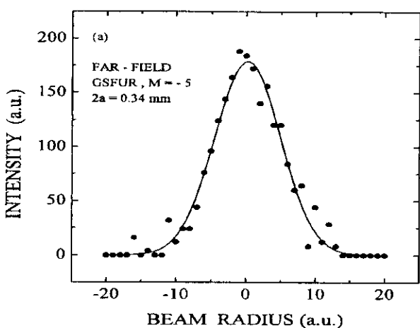
شکل ۴- نمونه‌ای از توزیع شدت میدان دور، اندازه‌گیری با مشاهده فلورسان صفحه مشاهده و آشکار سازی به وسیله دوربین CCD بوده است.
