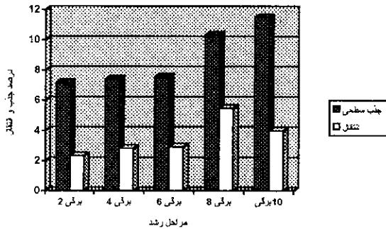
شکل ۳- مقایسه درصد جذب و انتقال سم 2,4-D از سطح برگ تلقیحی در مراحل پنج گانه رشد رویشی ذرت
