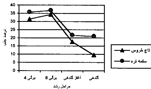
شکل ۱- مقایسه درصد جذب 2,4-D از سطح برگ تلقیحی طی مراحل رشد دو علف هرز
