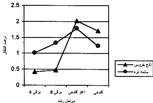
شکل ۲- مقایسه درصد انتقال 2,4-D به بالای محل تلقیح طی مراحل رشد دو علف هرز
