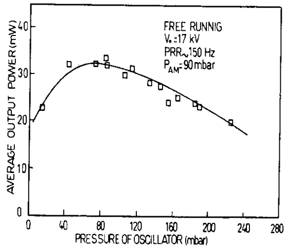
شکل ۱۰- نمودار تغییرات توان متوسط خروجی لیزر بر حسب تغییرات فشار گاز ازت در دستگاه نوسانگر، هنگامی که در گاف جرقه تخلیه آزاد صورت می گیرد. توان متوسط بدست آمده از سیستم در آهنگ تکرار ۱۵۰ Hz، برابر ۳۰ mW در ولتاژ ۱۷ کیلوولت بوده است.
