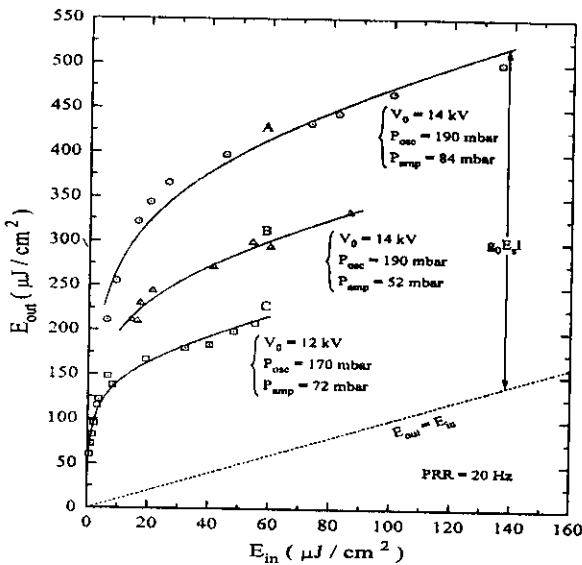
شکل ۹- نمودارهای نتایج اندازه گیری چگالی انرژی خروجی بر حسب تغییرات چگالی انرژی ورودی به دستگاه تقویت کننده در شرایط مختلف. نقاط اندازه گیری شده، مشخصه های کاری سیستم از جمله بهره سینگال کوچک، g_0 و چگالی انرژی اشباع E_S را بدست می دهند.
